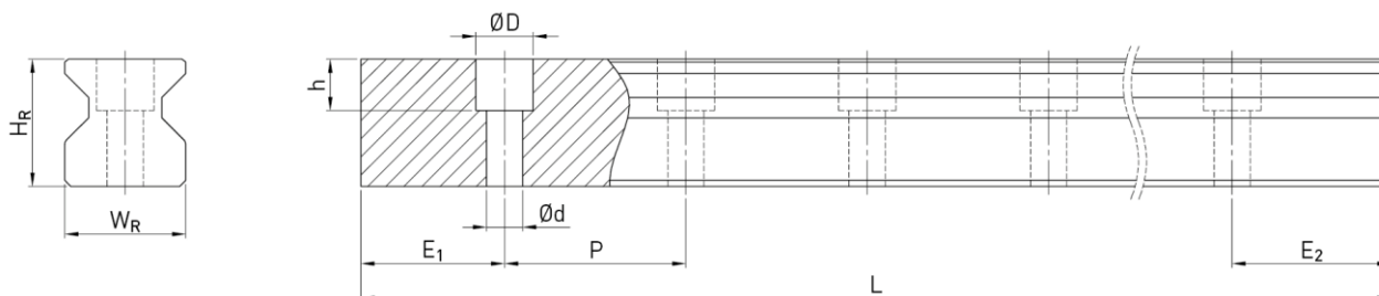
Rozměry kolejnice řady RGR_R
