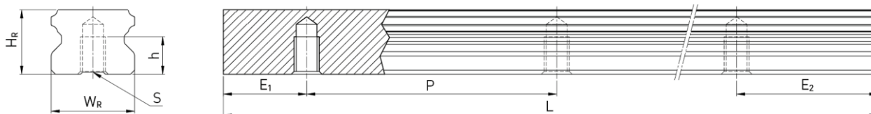
Rozměry kolejnice řady EGR_T
