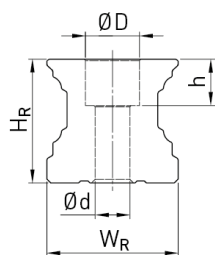
Rozměry kolejnice řady CGR_R
