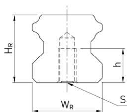
Rozměry kolejnice řady HGR_T
