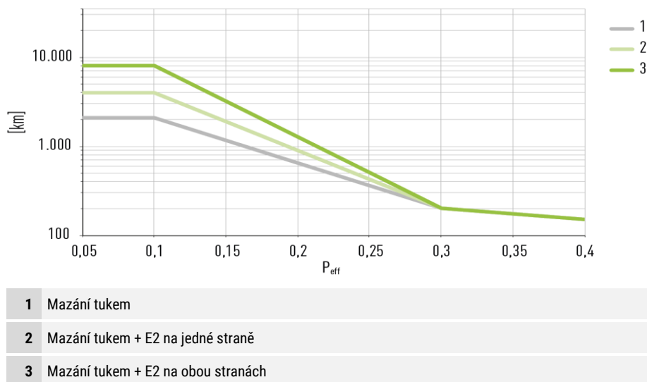
Obr. 8.23: Intervaly domazávání při mazání tuky, jednostranné a oboustranné jednotce dlouhodobého mazání (E2/EC) pro řadu UR a RG.
