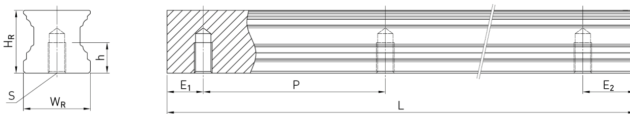
Rozměry kolejnice řady CGR_T
