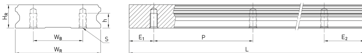
Rozměry kolejnice řady WER_T
