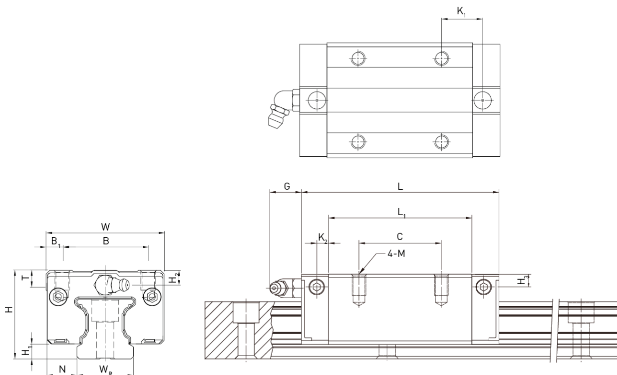
Rozměry vozíku
