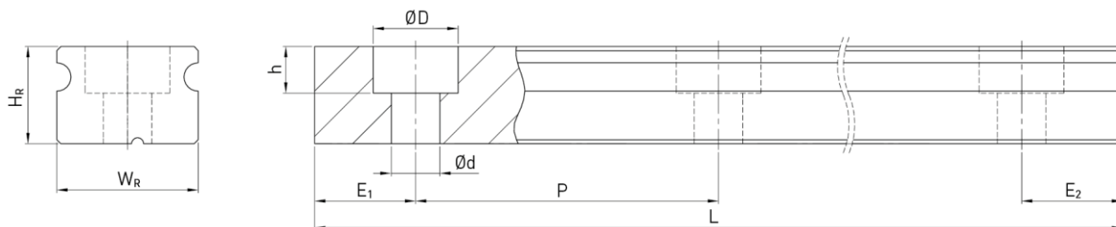
Rozměry kolejnice řady MGN_R
