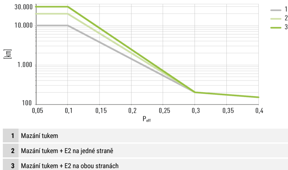
Obr. 8.22: Intervaly domazávání při mazání tuky, jednostranné a oboustranné jednotce dlouhodobého mazání (E2/EC) pro řady QH, QE a QW. Pro výrobní řadu QW není jednotka dlouhodobého mazání (E2/EC) k dispozici.
