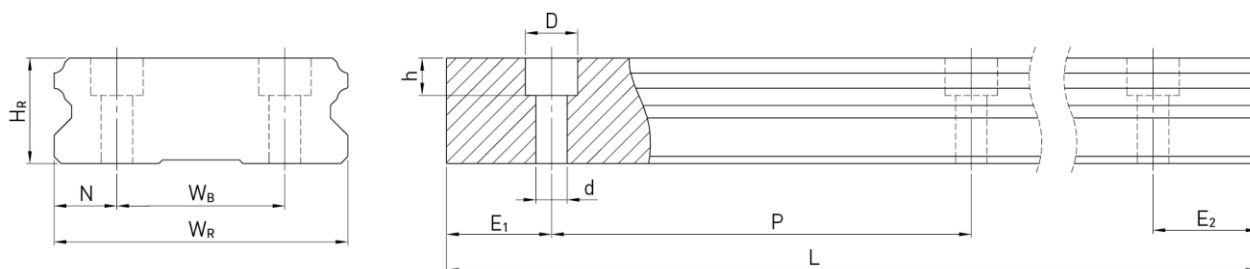
Rozměry kolejnice řady WER_R
